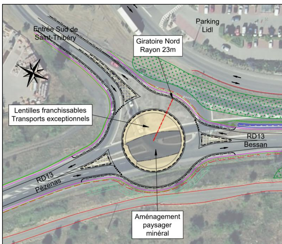
Plan de principe du giratoire d'entrée sud de saint Thibéry
