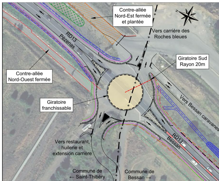
Plan de principe du giratoire d'accès à la carrière
